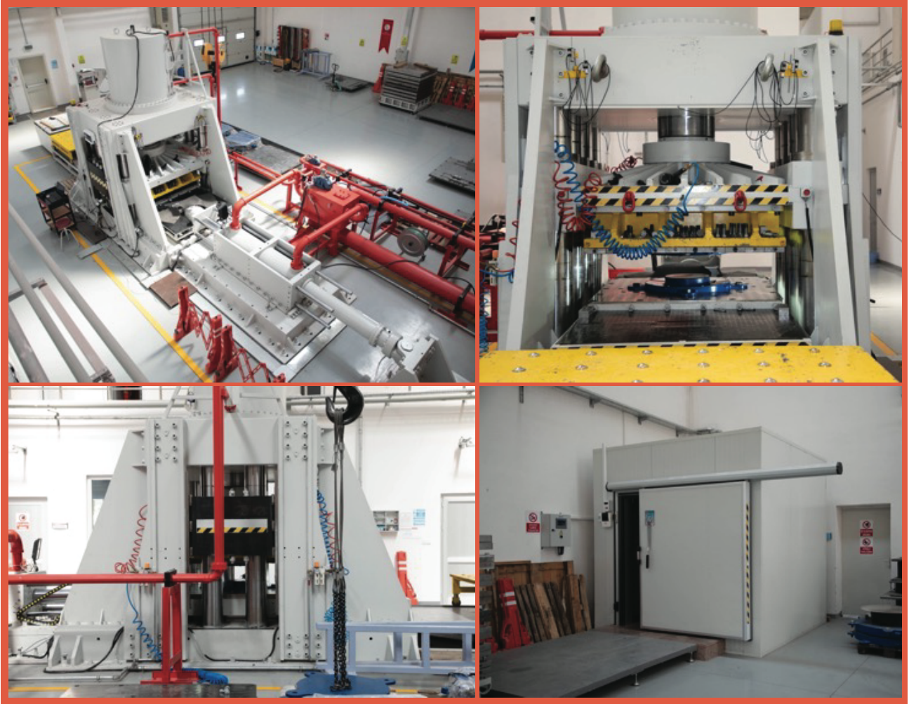
Şekil 1. ESQUAKE deprem izolatör test düzeneği
